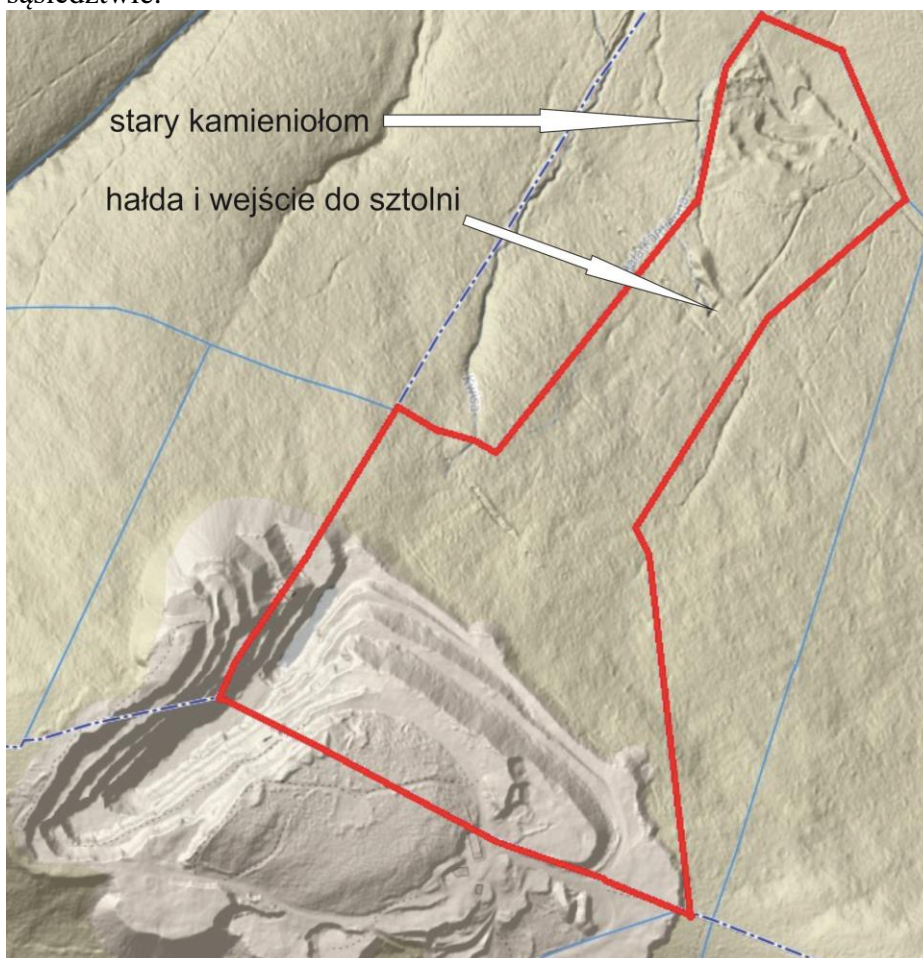
Rys. nr 2. Rzeźba terenu w zasięgu obszaru projektu Planu i w jego bezpośrednim sąsiedztwie.
